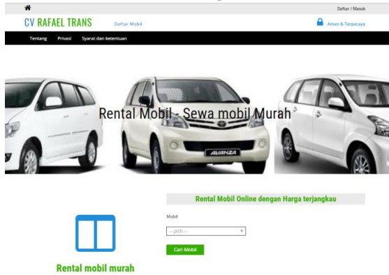
Gambar 15. Tampilan Utama
